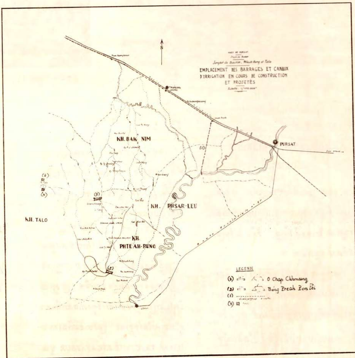
ផែនទីនៃទំនប់ទឹកដែលត្រូវធ្វើឱ្យសម្រេចឡើងក្នុងពេលឆាប់ៗនេះ
